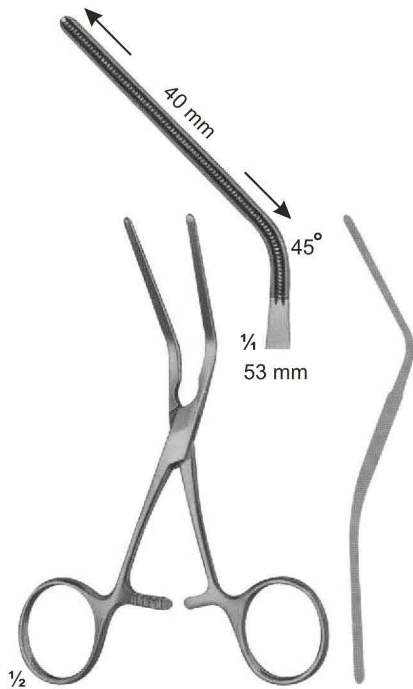
UG-1341 DE-BAKEY 45° winklig gebogen angled 45° 125 mm
