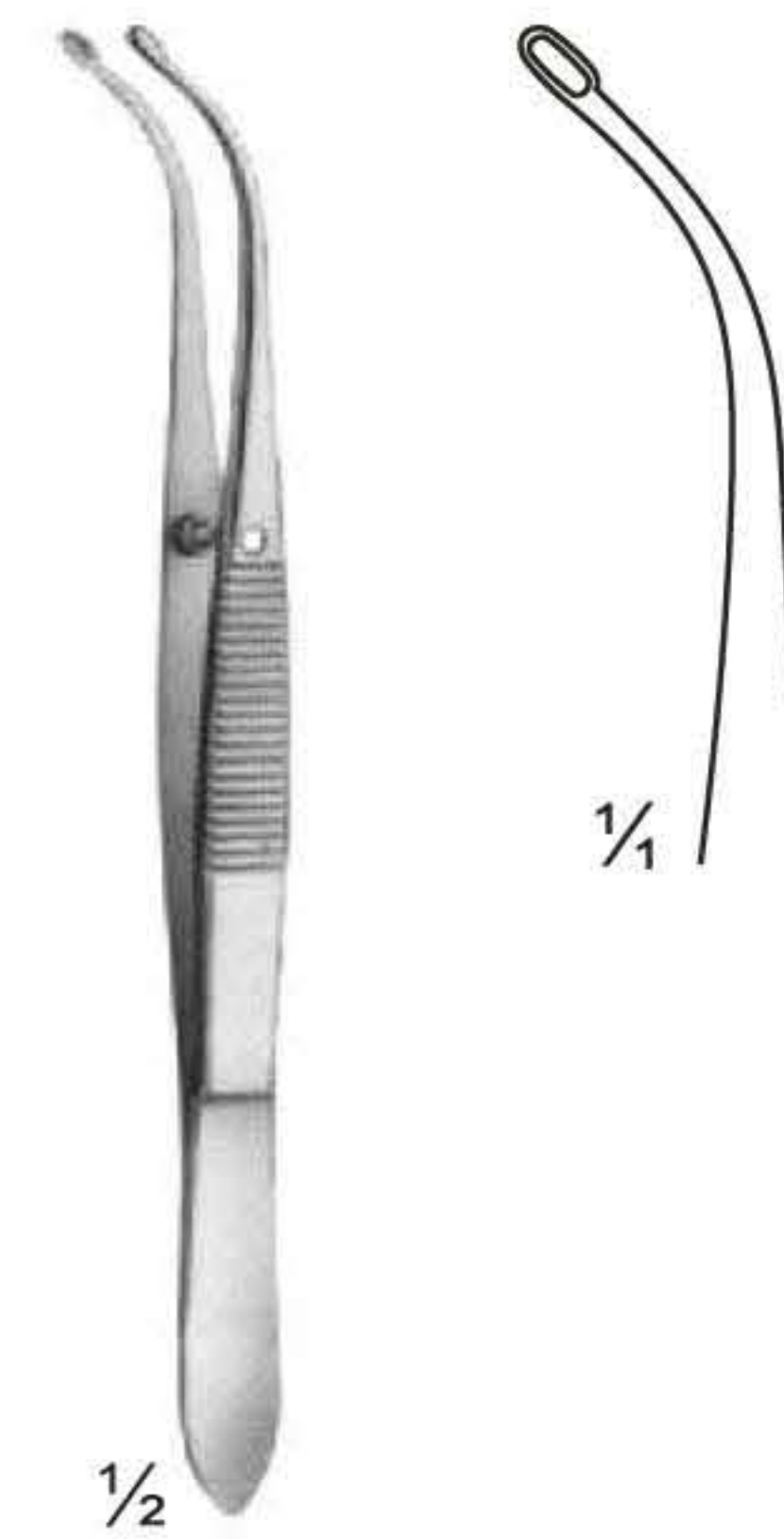
UG-250 ARRUGA 100 mm
